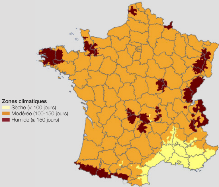
Nombre moyen annuel de jours de précipitations supérieures à 1 mm.
