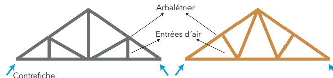
Figure 4 : Schéma de fermette de type « en M » en métal (gauche) et de type « en W » en bois (droite)
