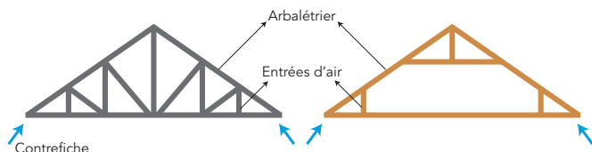
Figure 2 : Schéma de fermette de type « en N » en métal (gauche) et de type « à entrain retroussé » en bois (droite)
