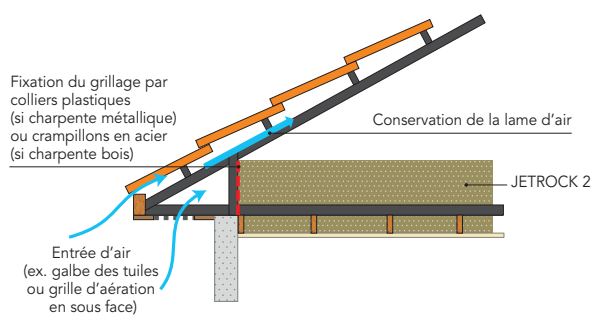
Figure 3 : Schéma de principe de la mise en œuvre du grillage de confinement sur une charpente industrielle métallique « petit entrain »
