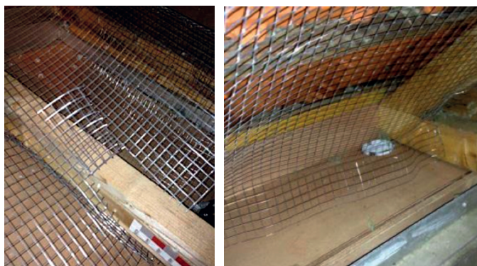
Figure 6 : Découpe et pliage du grillage en correspondance des entrainés (gauche) et maintien de l'aération (droite)
