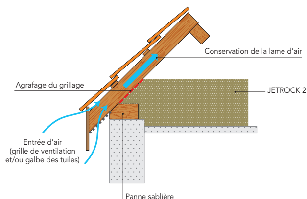
Figure 1 : Schéma de principe de la mise en œuvre du grillage de confinement sur une charpente traditionnelle
