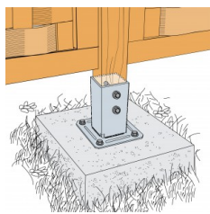
Fixation de clôtures sur support rigide
