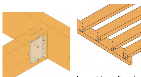
Assemblage discret sur poutres apparentes
